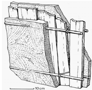
Abb. 3: Spalllattenkonstruierte Wand mit Lehmverputz 12
