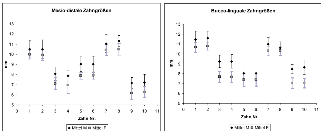
Abb. 11: Geschlechtsspezifische Zahngrößenunterschiede
