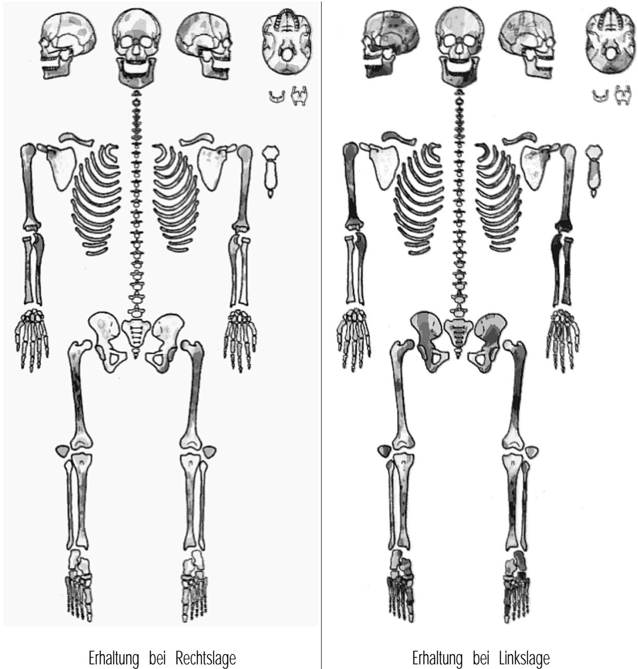
Abb. 10: Lageabhängige Erhaltungsunterschiede
