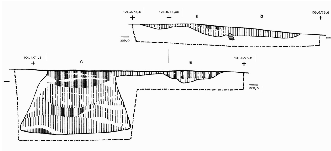
Abb. 95: Freiberg-Geisingen, LB, ‚Ried‘ (135c): Grubenkomplex 47. Profile. M. 1:40.
