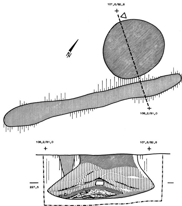
Abb. 87: Freiberg-Geisingen, LB, ‚Ried‘ (135c): Grube 25 und Schlitzgraben 26. Planum und Profil. M. 1:40.
